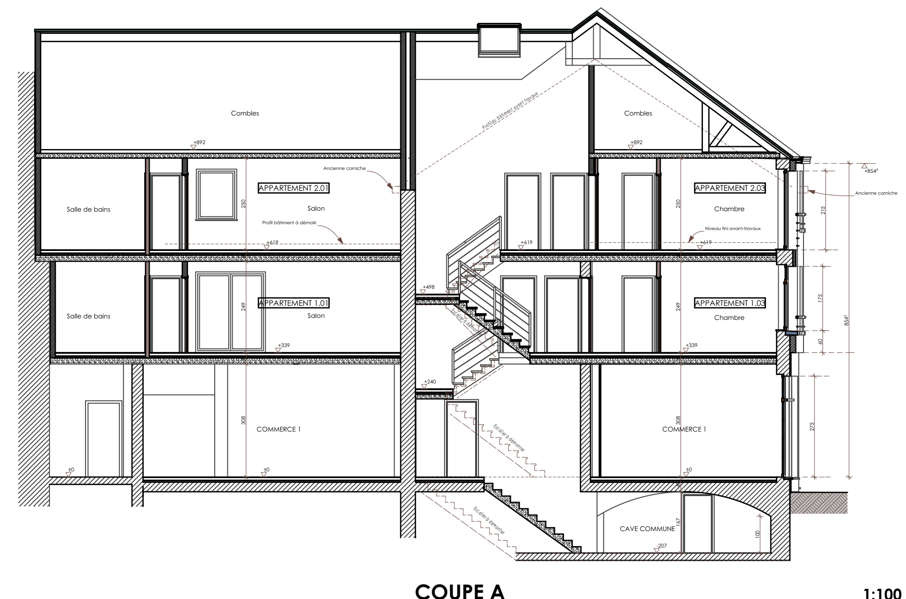
COUPE A 1:100
