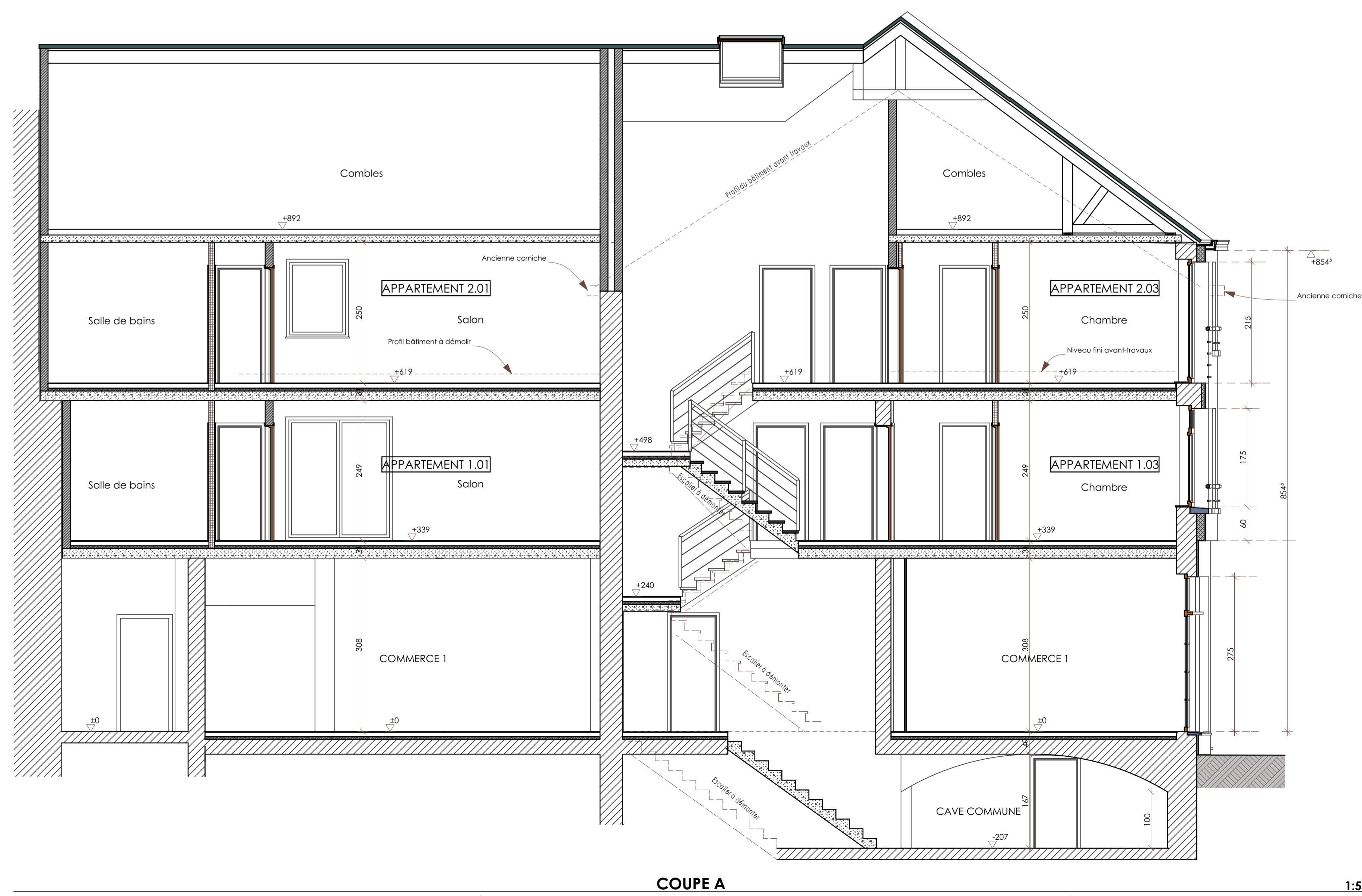
COUPE A
