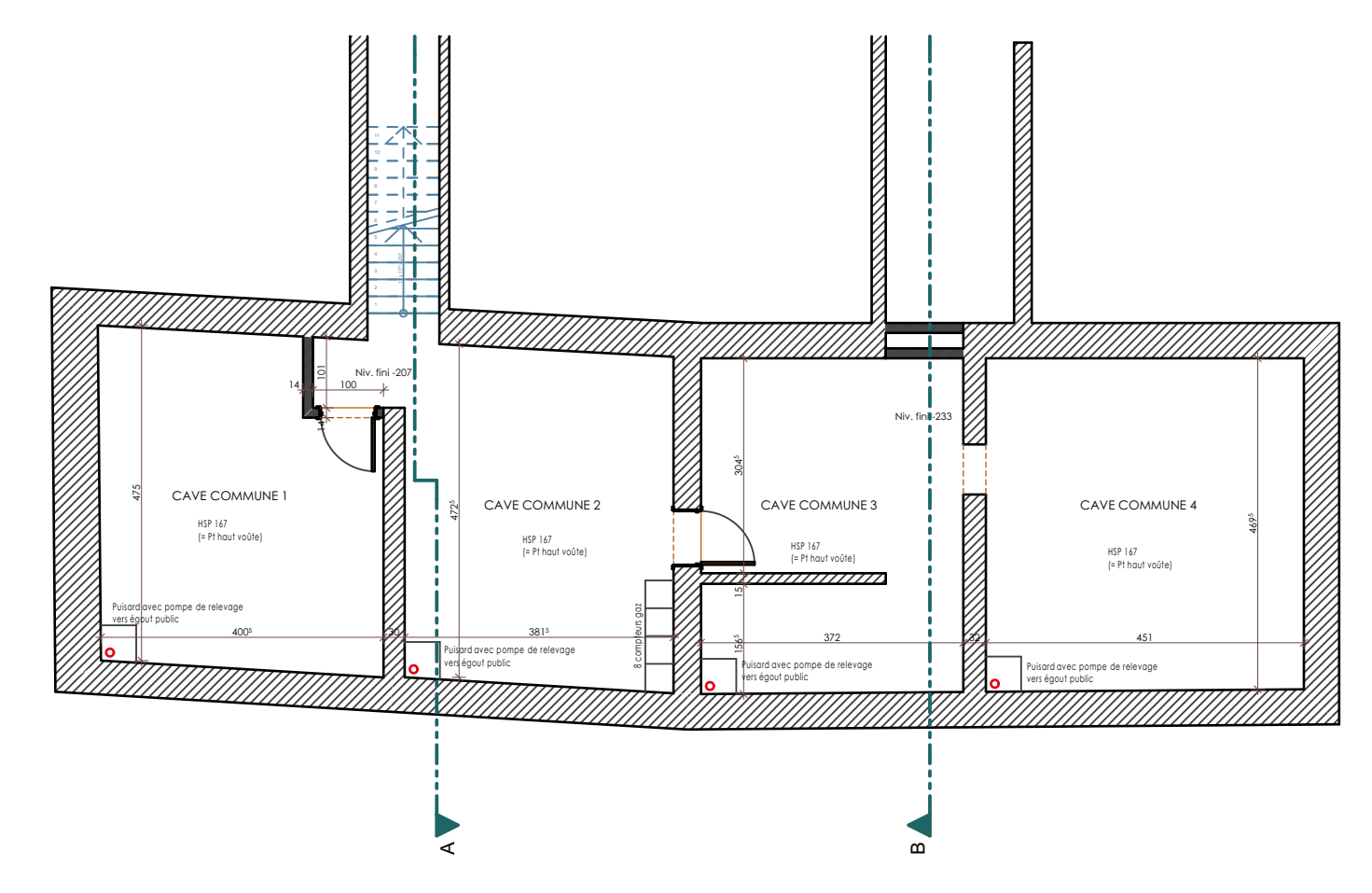
SOUS-SOL 1:100
