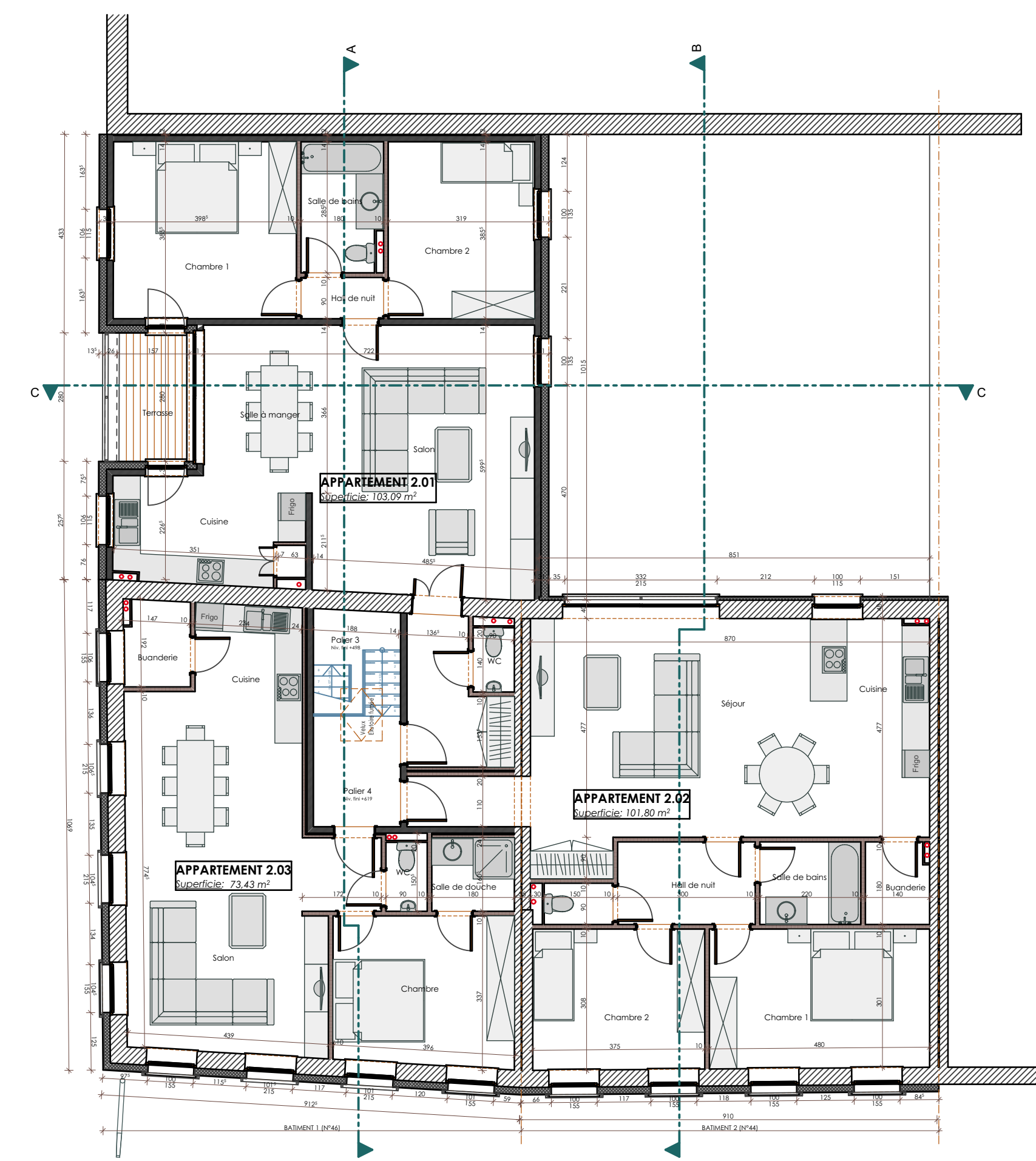
ETAGE 2 1:100
