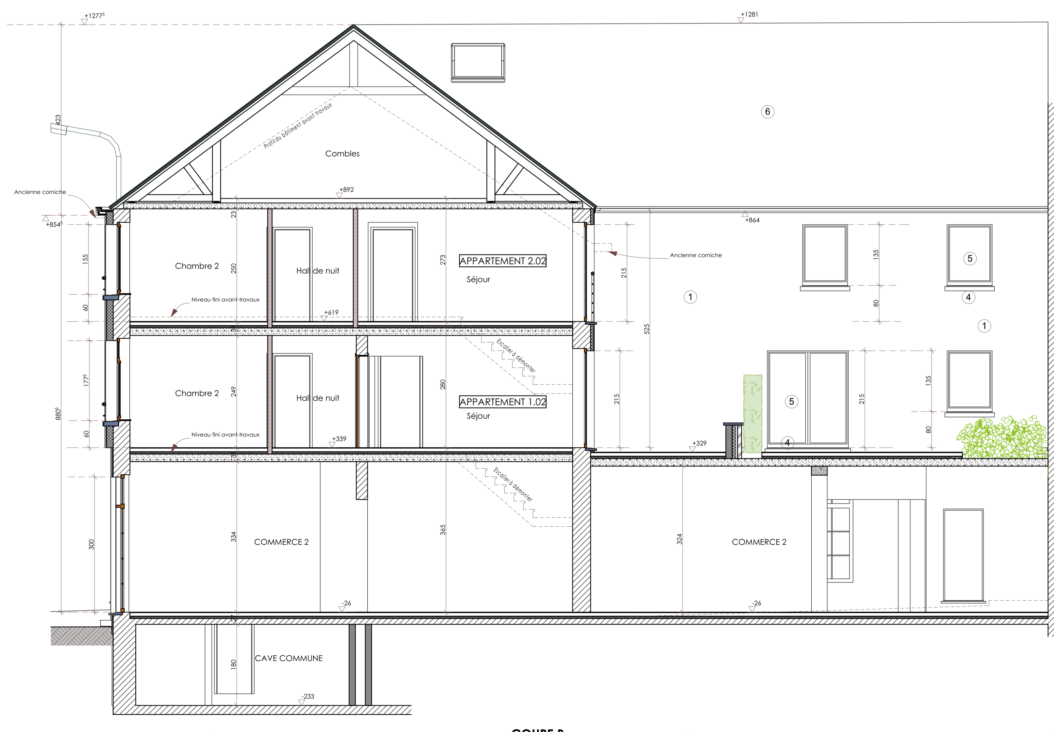
COUPE B
