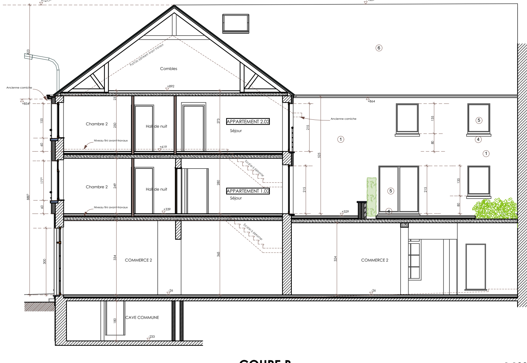
COUPE B 1:100
