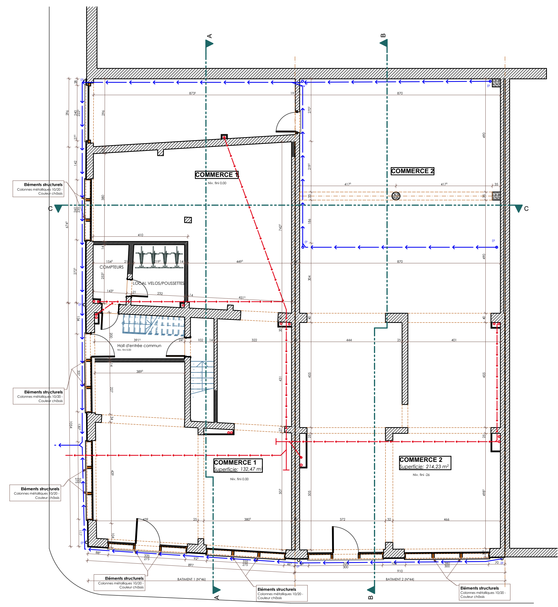
REZ-DE-CHAUSSEE 1:100
